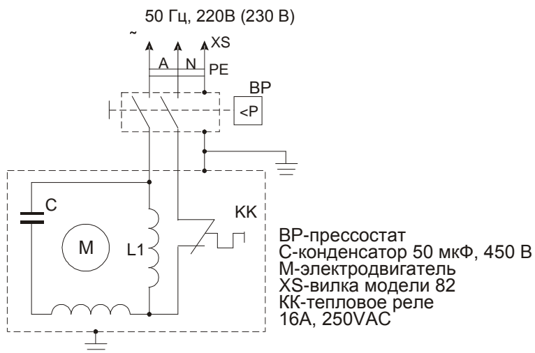
Рисунок А.1 - Схема электрическая принципиальная компрессоров СБ4/С-50.ЛВ24А, СБ4/С-100.ЛВ24А
