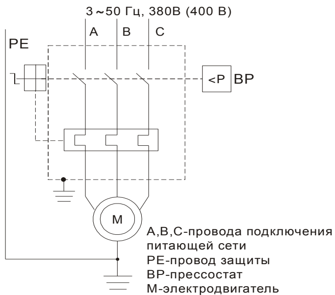
Рисунок А.2 - Схема электрическая принципиальная компрессоров СБ4/С-50.ЛВ24, СБ4/С-100.ЛВ24
